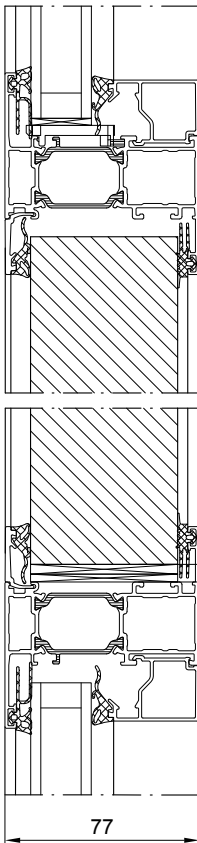
Schnitt B - B Section B - B
